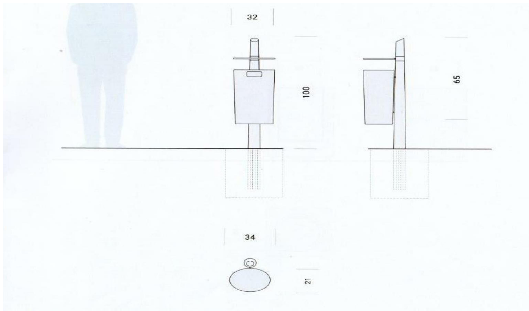
Слика4/ Мала ђубријера
