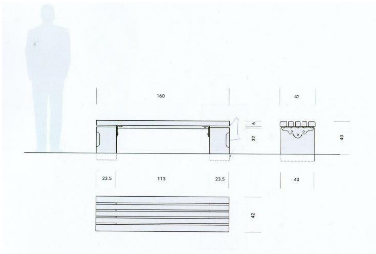
Слика 2/ Слободностојећа клупа
