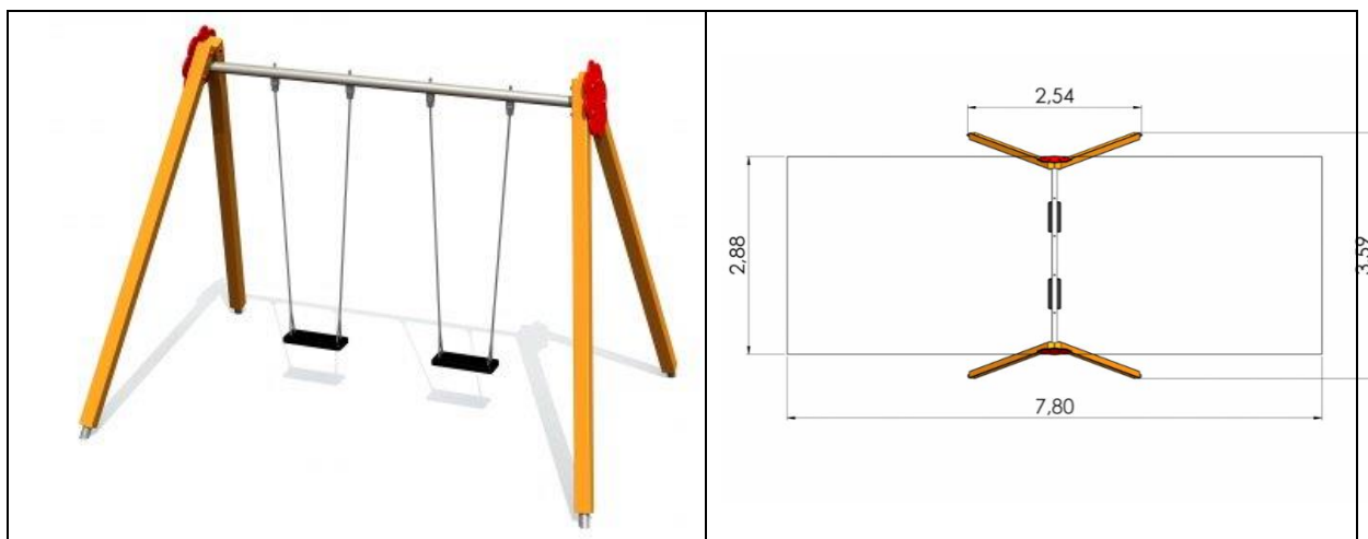
Скица 5. Љуљашка BELL-FLOWER 2 -konstrukcija
