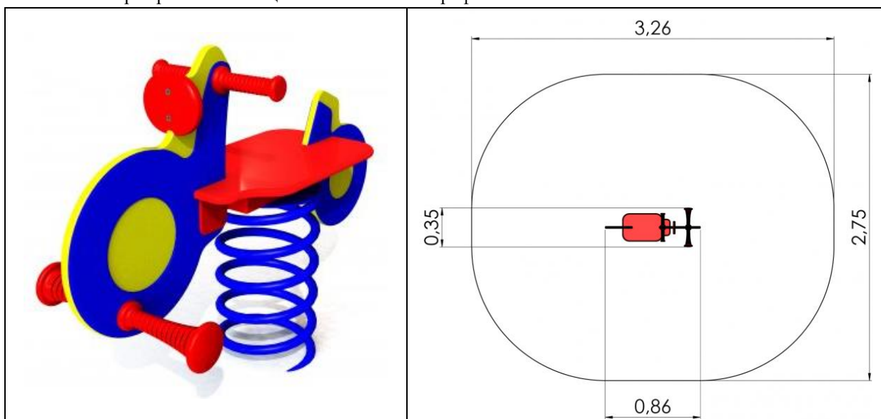
Скица 6. Њихалица Speedy
