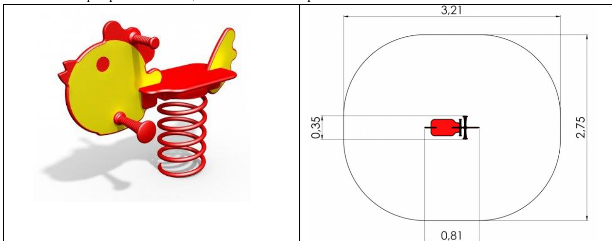
Скица 7. Њихалица TIBY
